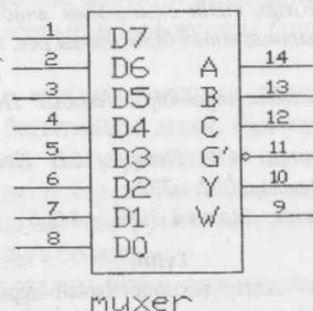
Сурет 1 – Мультиплексор
