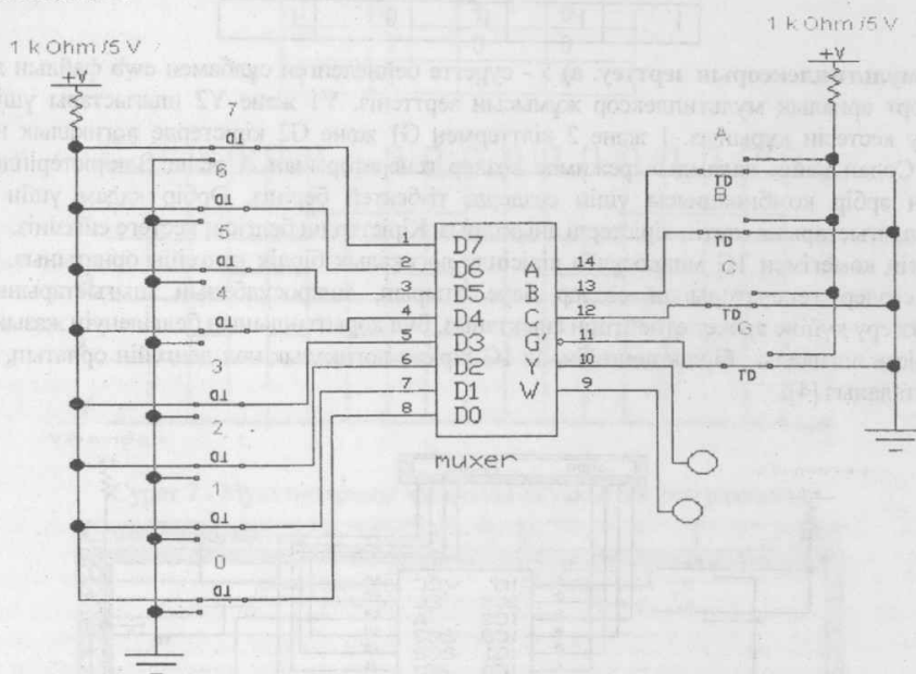
Сурет 4 - Мультиплексор сұлбасы
