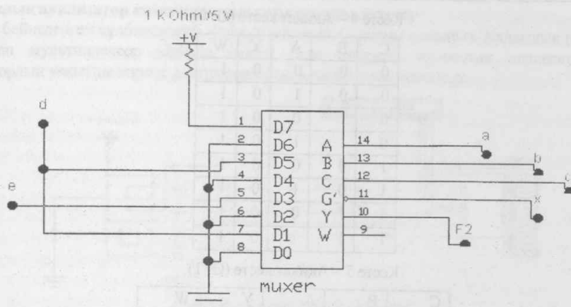
Сурет 3 - Мультиплексордың сұлбасы
