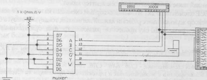
Сурет 6-мультиплексор сұлбасы
