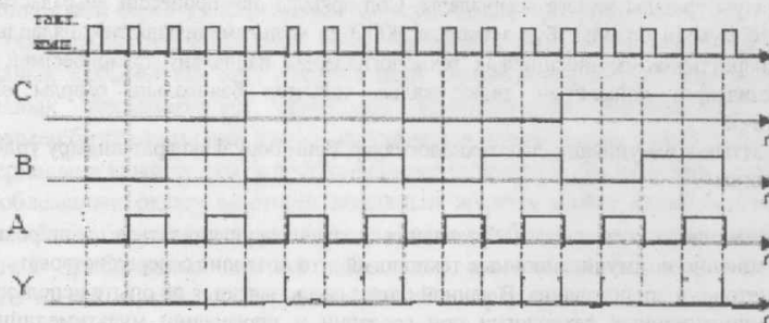
Сурет 7 - Мультиплексор жұмысының уақытша диаграммасы
