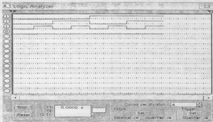
Сурет 8- Мультиплексор жұмысының уақытша диаграммасы (логикалық анализаторда)
