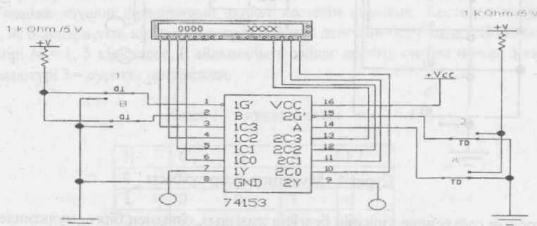
Сурет 5 - 74153 мультиплексорының сұлбасы
