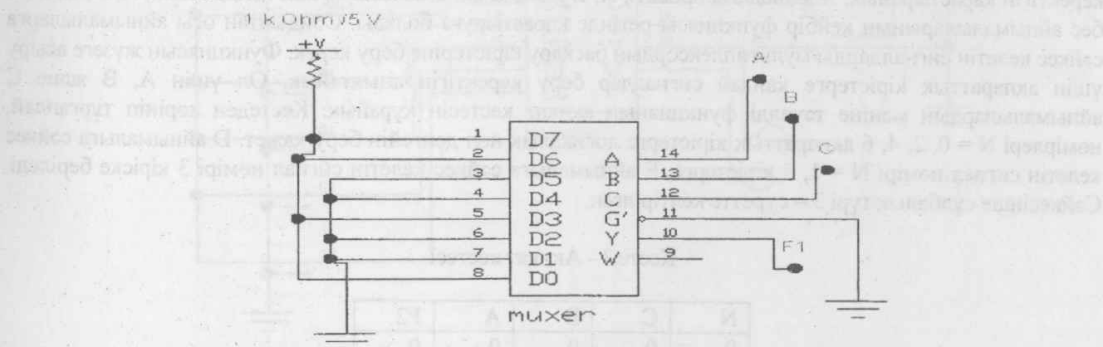
Сурет 2 – Мультиплексор функциясын жүзеге асыру сұлбасы
