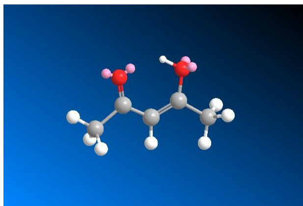
Рисунок 8 - Свернутый конформер № 3
