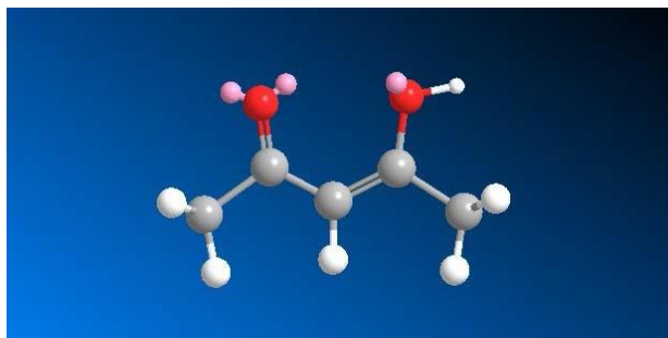
Рисунок 7 - Свернутый конформер № 2
