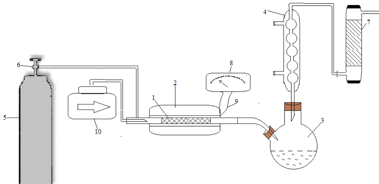
1 – проточный реактор, 2 – печь, подогреватель, 3 – приемник, 4 – холодильник, 5 – баллон с азотом, 6 – редуктор, 7 – вывод \text{H}_2 , 8 – вольтметр, 9 – термопара, 10 – система дозированной подачи реагентов
