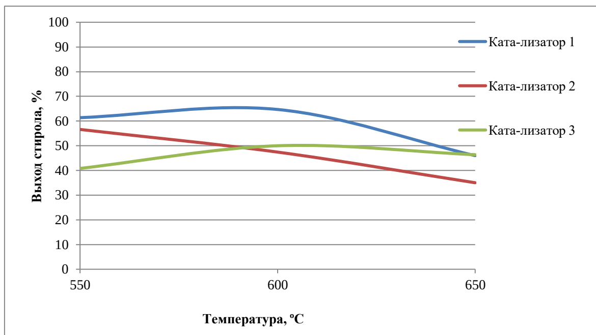
Рисунок 2 - Зависимость изменения выхода стирола от температуры реакции в присутствии катализаторов К-1, К-2 и К-3
