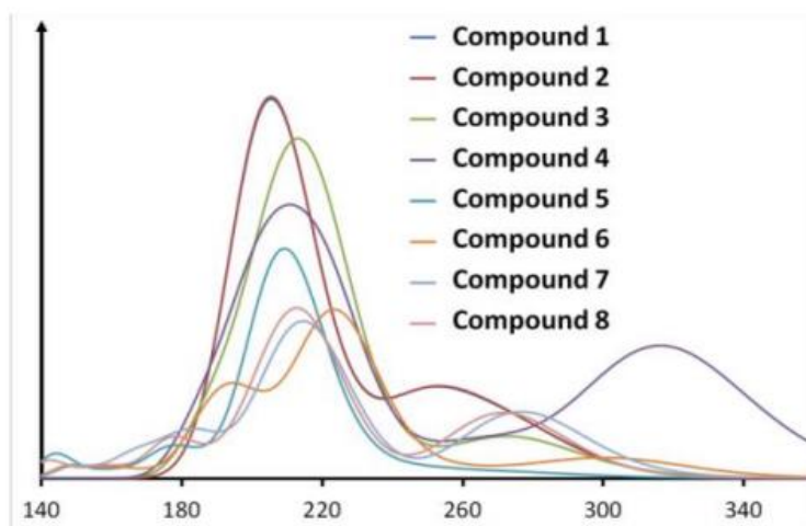
Сурет 4. ZINDO әдістерін қолдана отырып, жоғарыда аталған сегіз қосылыстың болжамды ультрафиолетті спектрлері
