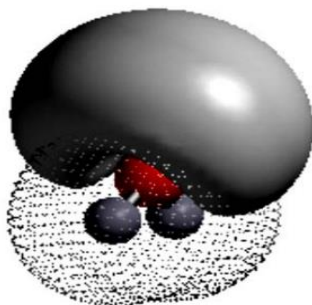
Сурет 5. Еркін электронды жұпты, сондай-ақ Ван-дер-Ваальдарды сүтегі атомдарының радиусын көрсететін су молекуласының 3D моделі
