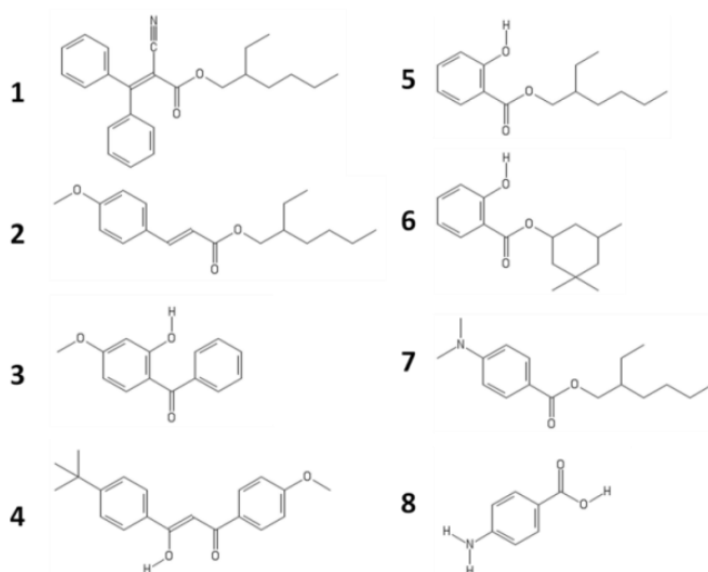
Сурет 3. Біріктірілген \pi -жүйемен қосылыстар sunscreen жобасы аясында зерттеу
